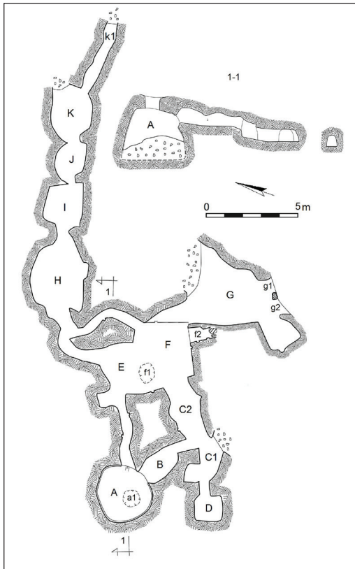
איור 7: מערכת המסתור, תכנית וחתך 1-1
